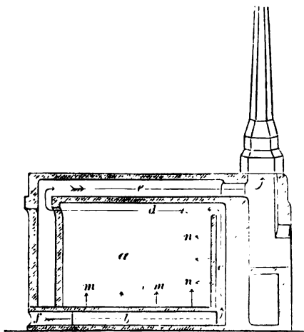
Č. 1810. Pec kasselská.
